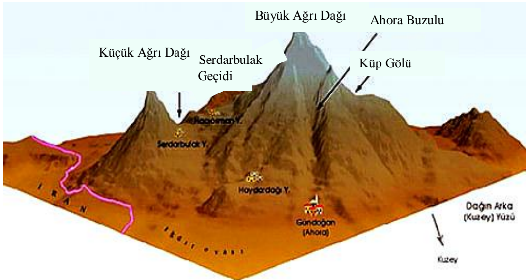
Resim 1: Büyük Ağrı Dağı ve Küçük Ağrı Dağı'nın Kabartma Resmi 8
