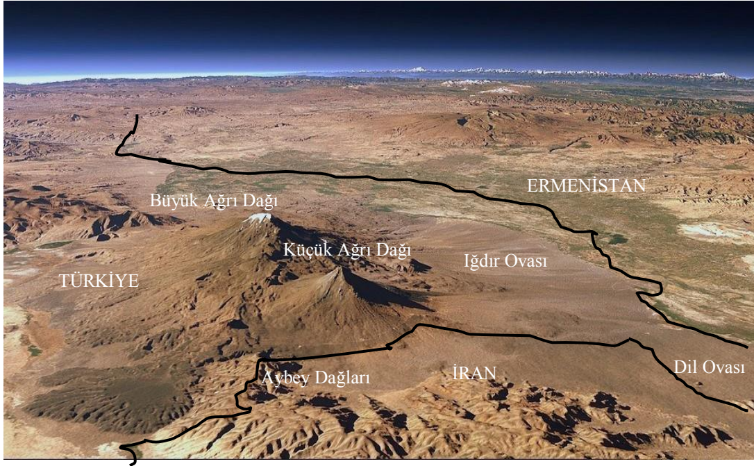
Fotoğraf 1: Büyük Ağrı Dağı ve Küçük Ağrı Dağı'nın Uydu Fotoğrafı 10
